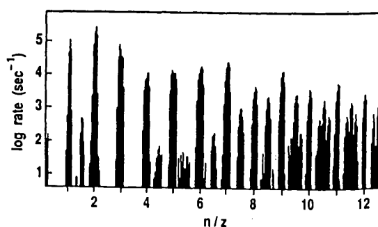
図4 液体金属イオン源で生成された金クラスターのサイズ分布。2価クラスターは 9^{++} から3価クラスターは 26^{3+} 以上で観測された。（文献3より）
