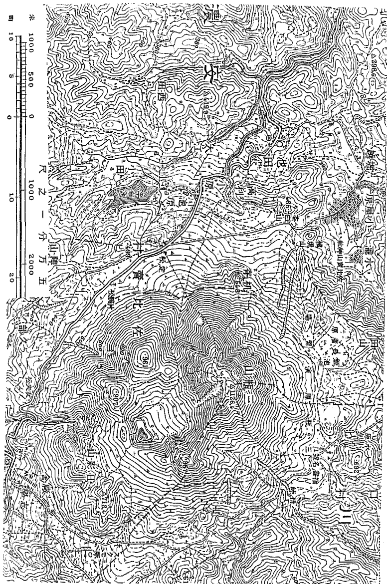
第二圖 三瓶火山の構成様式と地形 (陸地調査部地形圖)
