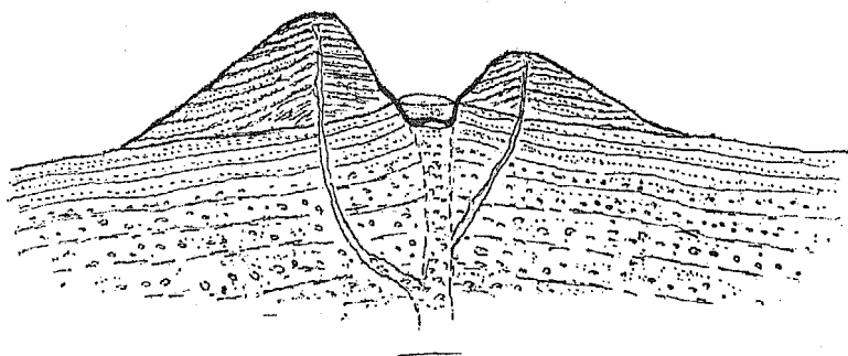
第三圖 三瓶火山構成様式 (室ノ内 細線は過去 太線は現在)
