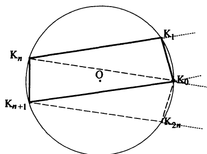
図 2.9: 正 m 角形の等脚台形 ( m odd)
