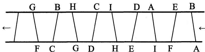
図 2.6: 正九角形を作るテープ (右から左へ見て下さい)
