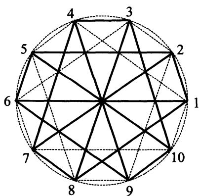
图 2.12: 正十边形 ( \frac{m}{2} odd)
