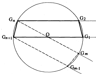
図 2.10: 正 m 角形の等脚台形 ( m even)
