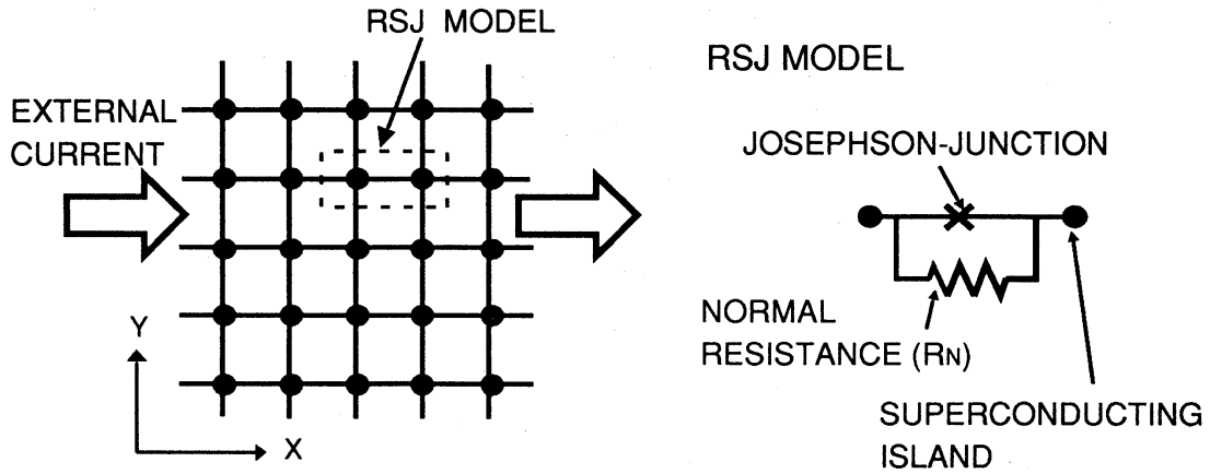
図 3. RSJ Model.
