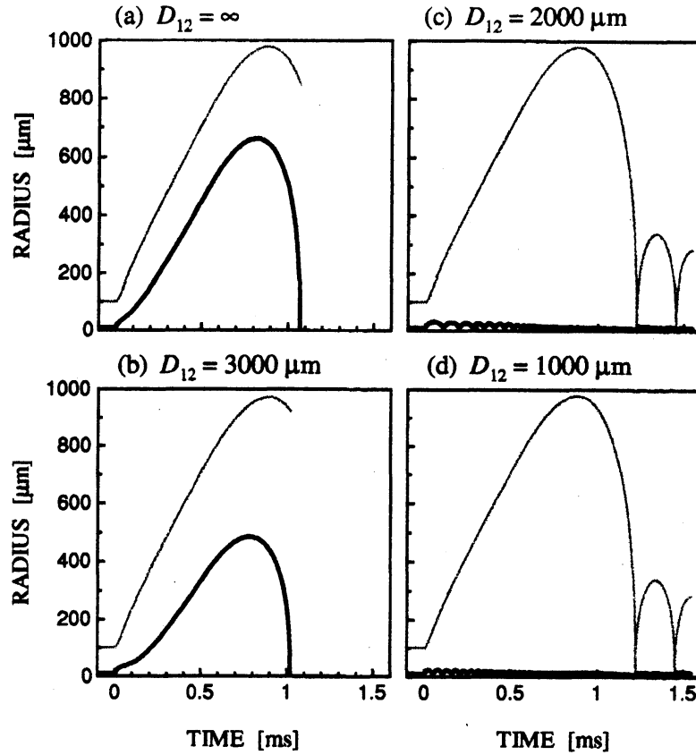
Fig. 5. 異なる D_{12} に対する二気泡系 ( R_{10}=10 \mu\text{m} 、 R_{20}=100 \mu\text{m} ) の半径変化。太線はキャビテーション気泡、細線はヘリウム気泡を表す。 D_{12} \geq 3000 \mu\text{m} の場合に観測されるキャビテーション気泡の急膨張が、 D_{12} \leq 2000 \mu\text{m} の場合にはヘリウム気泡によって抑え込まれている。
