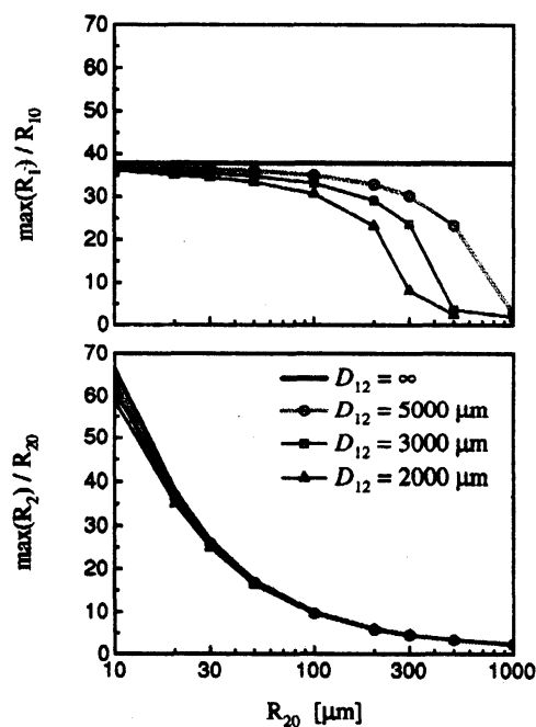
Fig. 8. Fig. 7 に同様。ただし、 R_{10} = 20 \mu\text{m} 。
