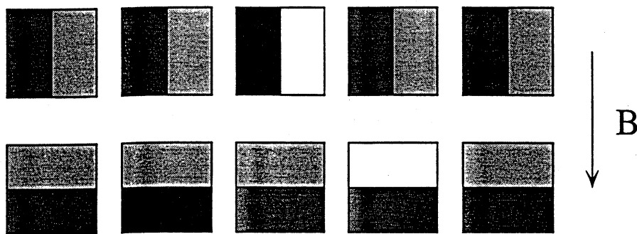
図1: 多重パイコね変換 B
