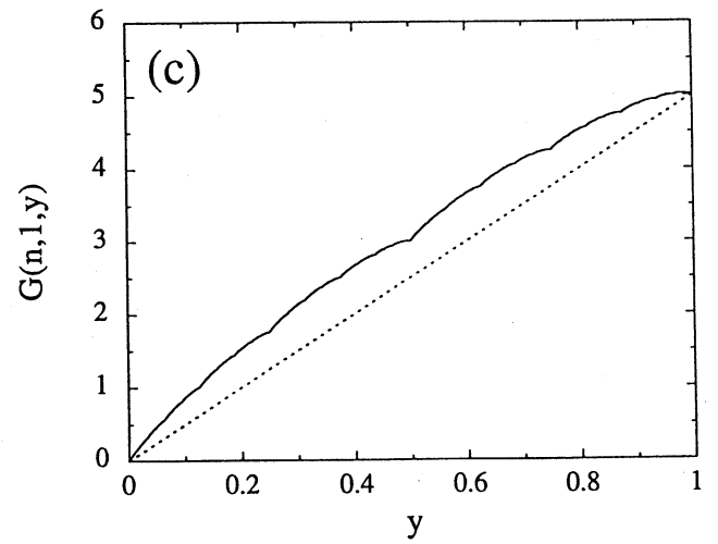
図 3 : 累積分布 G(n, x, y) のふるまい (\alpha = 1/2, \text{Fick 状態}) (a): G(n, 1, 1) v.s. n , (b): G(5, x, 1) v.s. x , (c): G(5, 1, y) v.s. y
