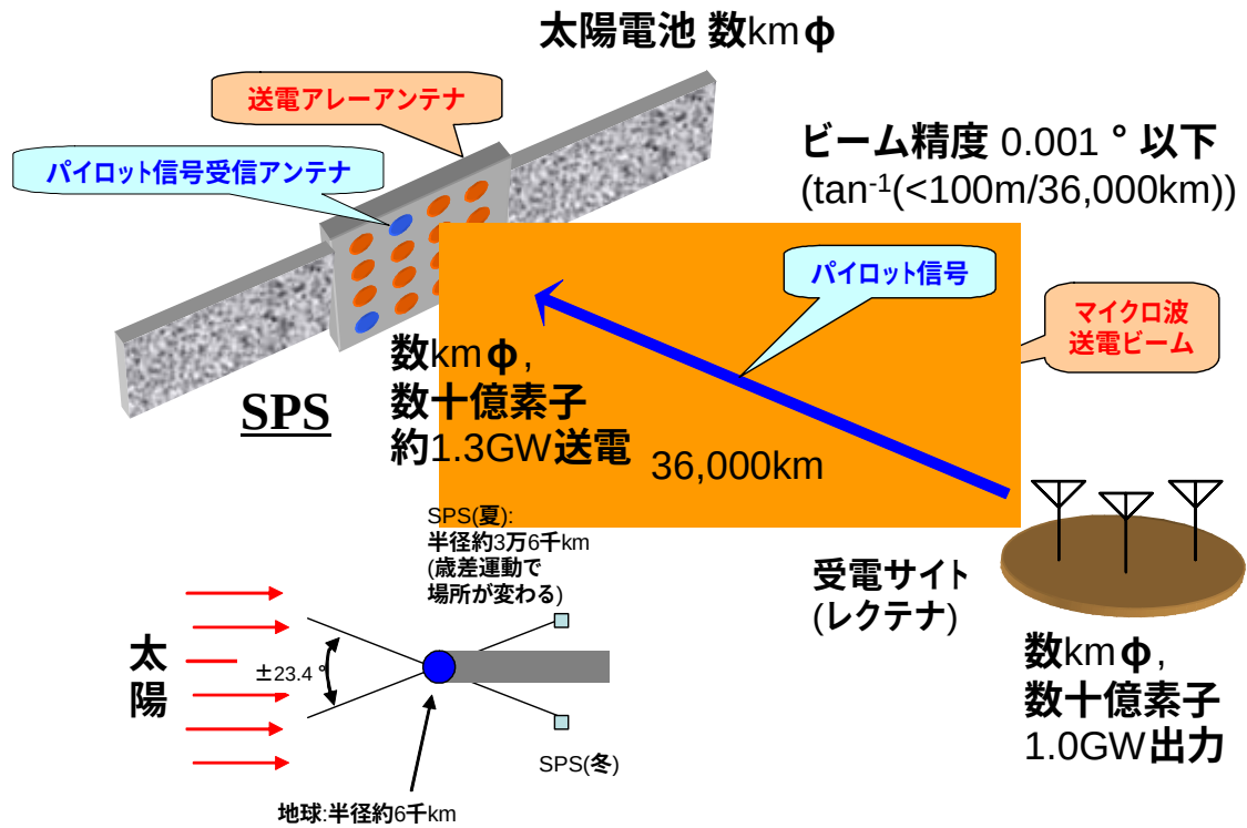
図1 SPS の一般的な概念とパラメータ
