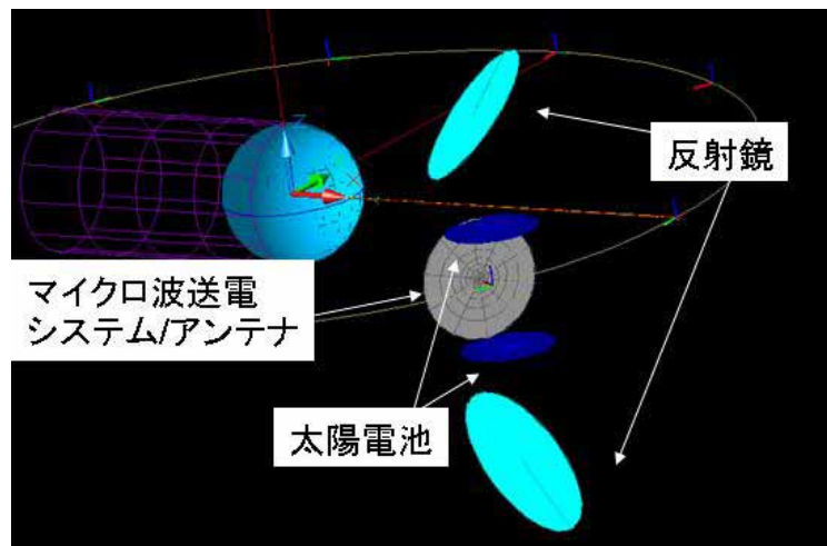
図2 JAXA-SPSの概念図 (2004年モデル) 一次ミラー：2.5km×3.5km, 1,000 t×2, 発電部：1.2km～2kmφ(TBD), 送電部：1.8～2.5kmφ, 発電部と送電部をあわせて8,000t程度 [9]
