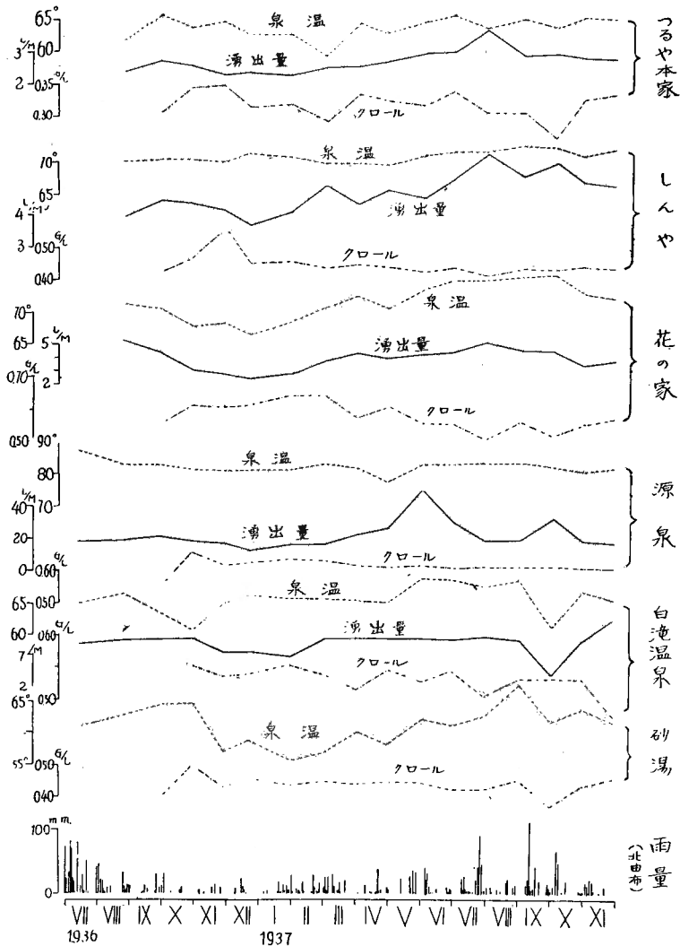
第2圖 湯平溫泉：湧出量、泉温及クロール量變化
