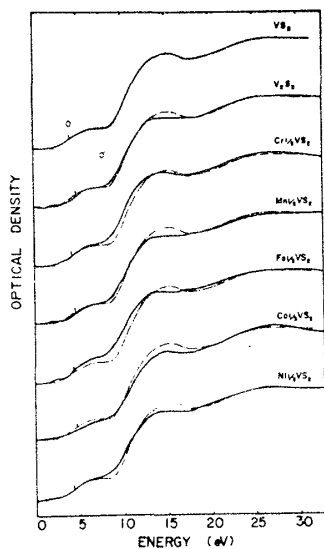
図5. M_3VS_2 のV-K吸収スペクトル 一点鎖線は母体のスペクトルを示す。
