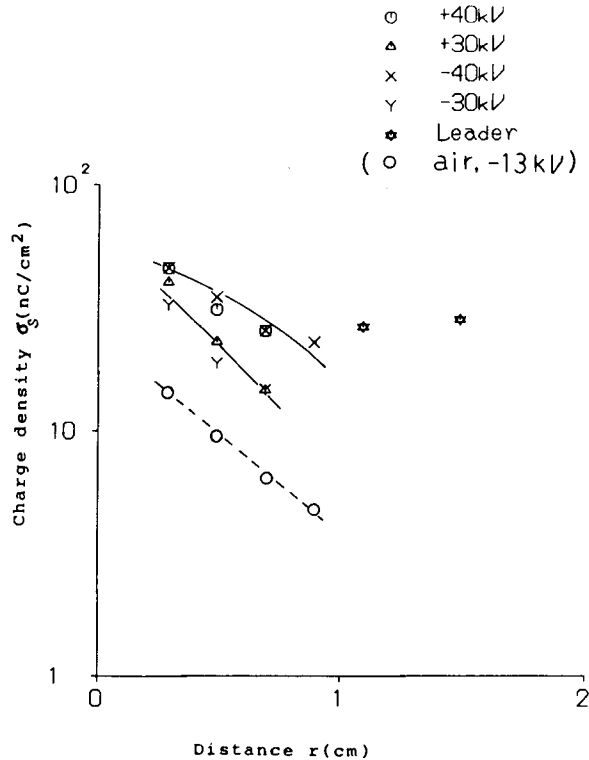
(a) 1.0 atm SF_6 .
