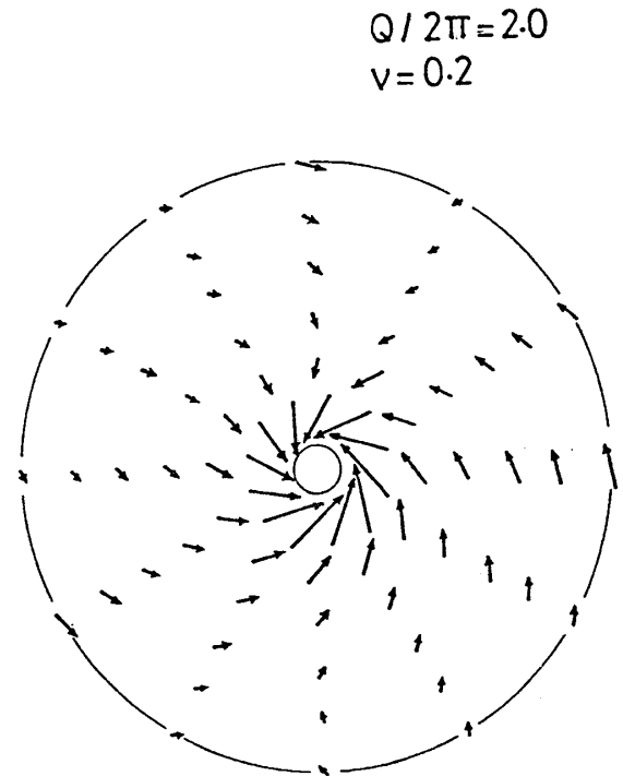
図3 計算機シミュレーションによる渦のパターン。
