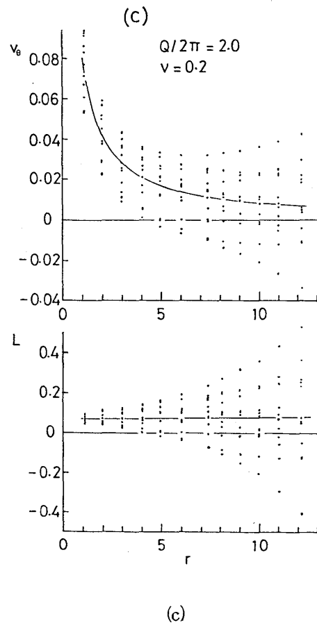
図4 計算機シミュレーションによる v_\theta および L の分布
