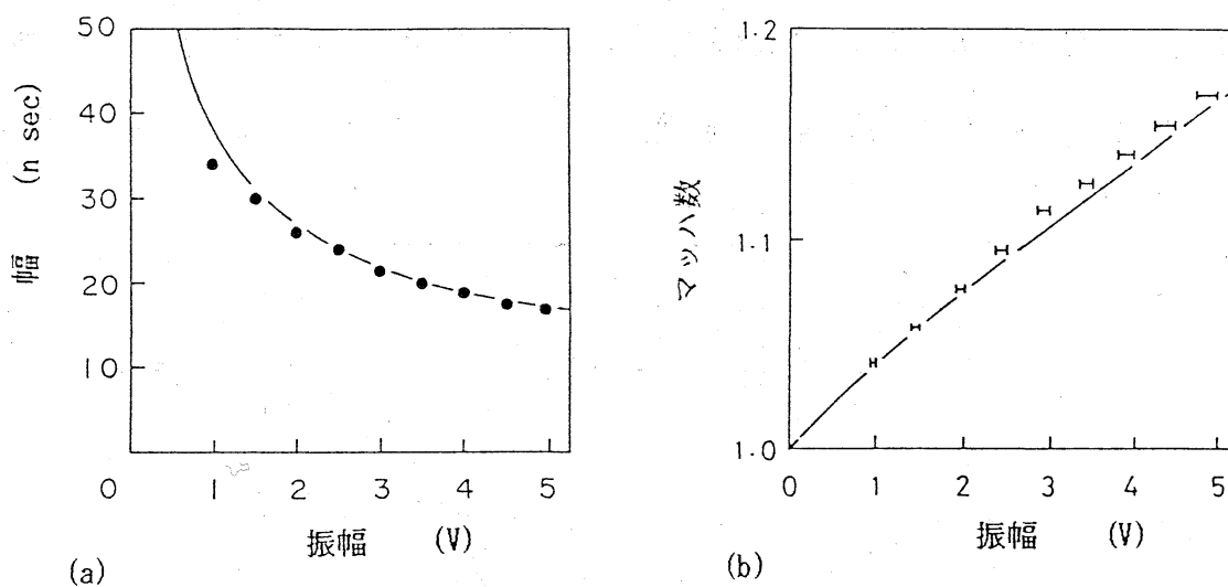
図7 ソリトンの幅(a)と速度(b)
