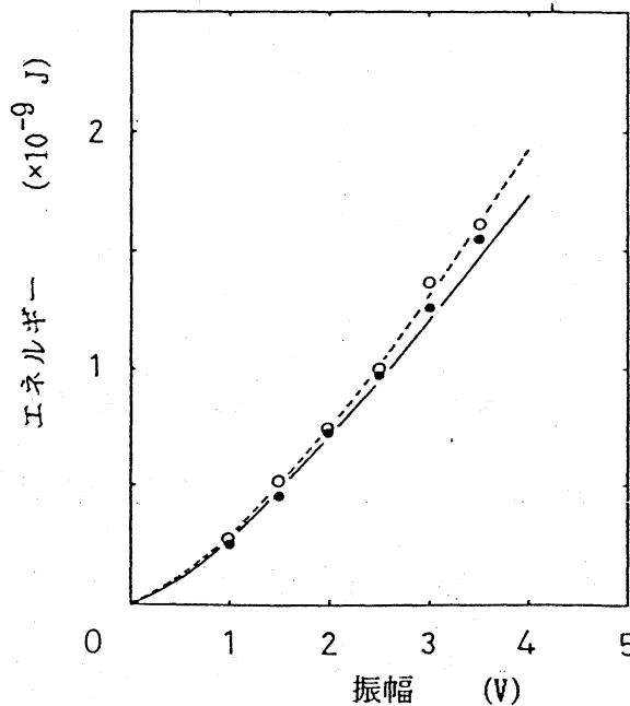
図8 ソリトンのエネルギー
