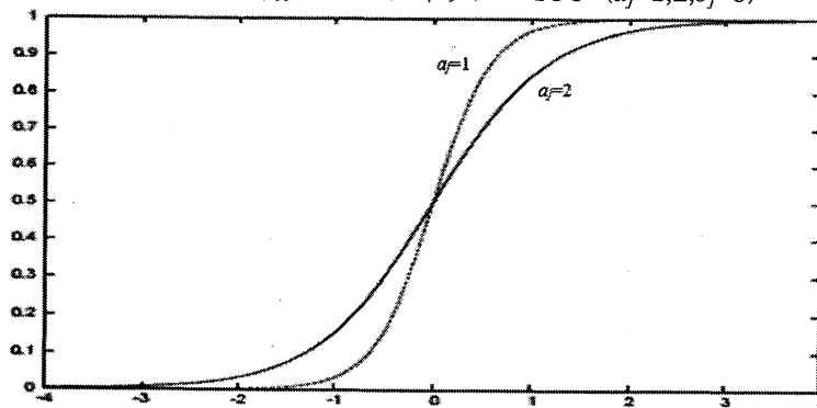
グラフ 2.2 2-母数ロジスティックの ICC ( a_j=1,2, b_j=0 )
