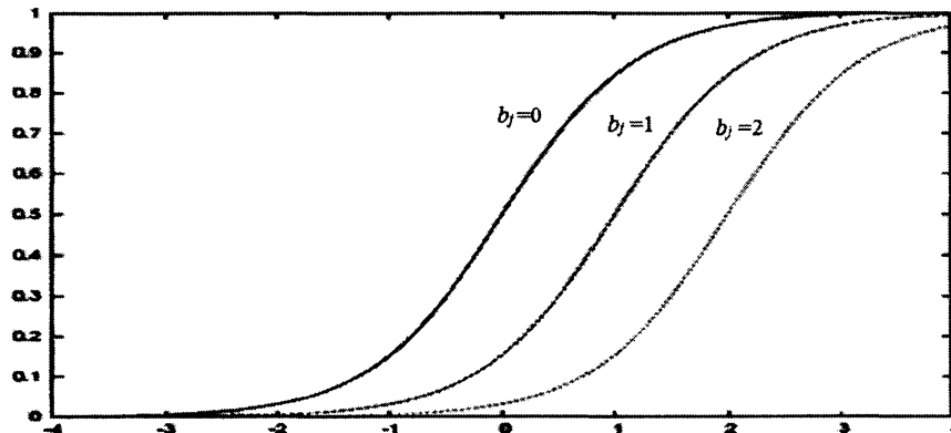
グラフ 2.1 1-母数ロジスティックの ICC ( a=1, b_j=0, 1, 2 )
