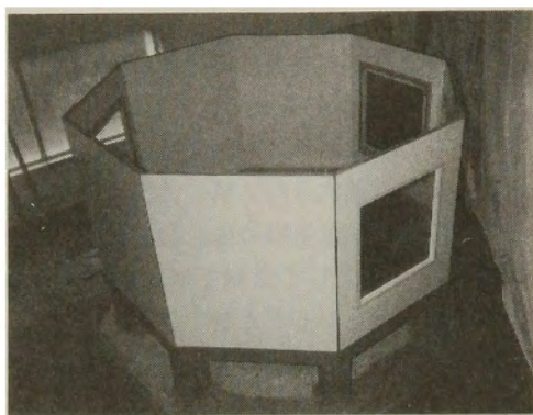
写真4 仮組立てのあと各コーナーにシリコン打ち。
