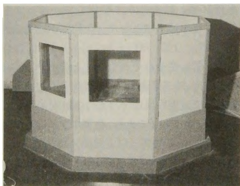
写真5 塩ビ製の枠とスカートを取付け完成。
