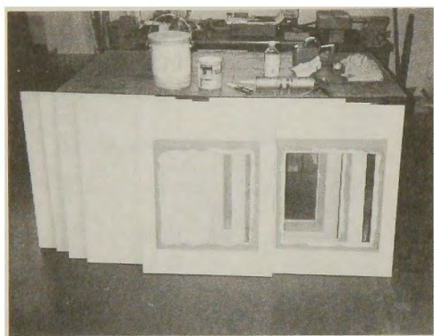
写真2 新321号水槽側面板、内4枚にガラスを接着。
