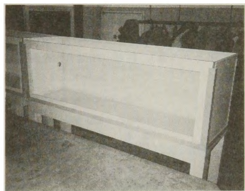
写真 7 組立て：塩ビ枠で仮止め シリコン打ち。
