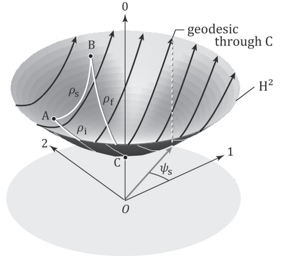
Fig. 6. Schematic illustration for the isometry (solid arrows) on H^2 corresponding to pure shear. Gray arrows are the orthogonal projections of the solid arrows onto the 12-coordinate plane. The azimuth of the gray arrow relative to the 1-coordinate axis is equal to \psi_s . The white line on H^2 depicts the hyperbolic triangle with vertices, A, B and C, shown in Fig. 1. 実空間における純剪断に対応した H^2 上の等長変換を表す黒い太線の矢印。その第 12 座標平面への正射影は平行線になる。Fig. 1 の双曲三角形が H^2 上の白線で表されている。
