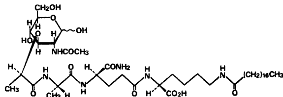
MDP-Lys(L18); muroctasin
