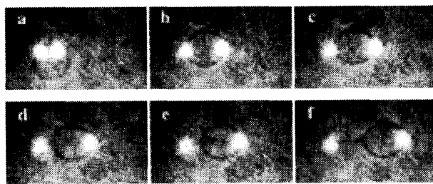
図1 光ピンセットを用いたビーズによるリポソームの突起形成。 縮尺：10 \mu\text{m}
