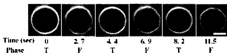
図3 リポソームの繰り返し振動
