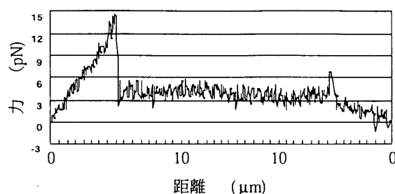
図2 膜突起形成・伸長・短縮に必要な力。突出時に最大の力が要り、伸長時は小さな力で十分である。
