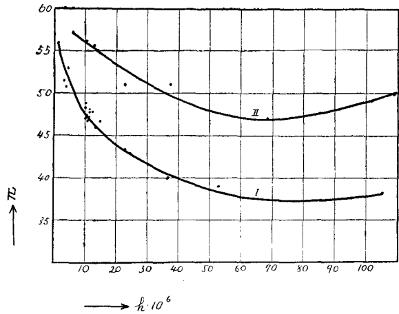
第一圖 硫安溶液内に於ける Ovalbumin の滲透壓に及ぼす水素イオンの濃度及硫安の濃度の影響 (Prof. Sørensen による)
