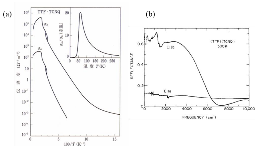
図 3 TTF・TCNQ における (a)伝導度の温度依存性と(b)反射率の波数依存性[2]。
