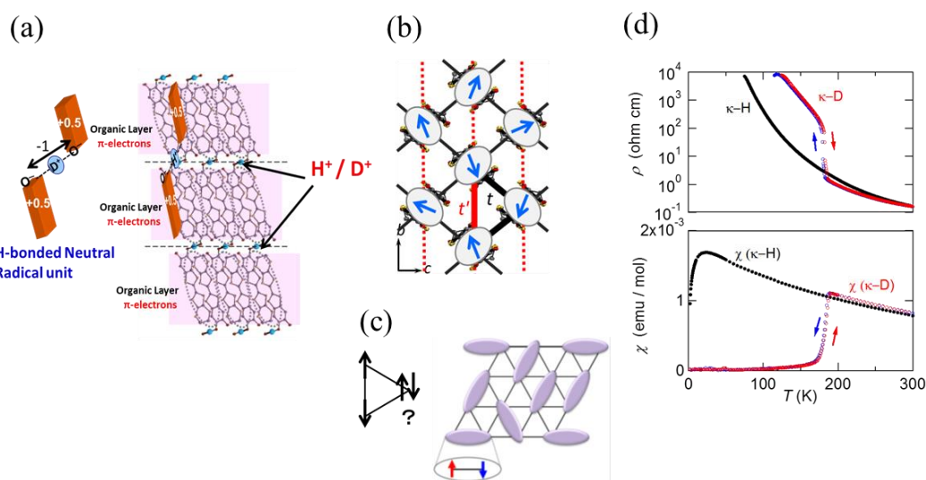
図7 水素結合プロトンと \pi 電子がカップルした新しい有機伝導体 \kappa\text{-X}_3(\text{Cat-EDT-TTF})_2 [ X = \text{H}, \text{D} ] では、(a)絶縁性アニオン層がなく、伝導層が水素結合 [(\text{O} \cdots \text{H} \cdots \text{O})^{1-}] あるいは [(\text{O} \cdots \text{D} \cdots \text{O})^{1-}] で連結された単成分純有機伝導体であり、(b) 伝導層は二量体分子が三角格子を形成したスピンのフラストレーション系となっており、(c) スピン対が量子的に共鳴する量子スピン液体を実現している。[9] (d) 水素結合のダイナミクスにより、水素体は量子スピン液体であるが、重水素体は 185K で磁性と伝導性のスイッチングが起こる。[6-8]
