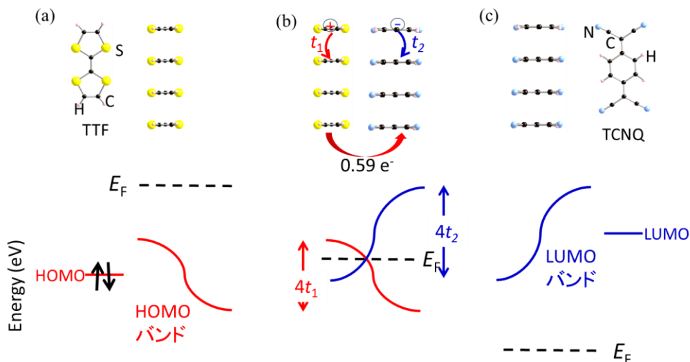
図 2 (a) 電子供与体 TTF の HOMO (the highest occupied molecular orbital) と HOMO バンド、(b) 電荷移動錯体 TTF・TCNQ、(c) 電子受容体 LUMO (the lowest unoccupied molecular orbital) と LUMO バンド。
