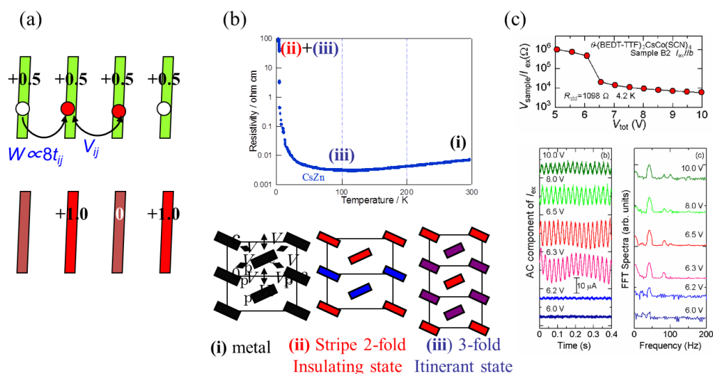
図6 3/4 充填バンドを有する強相関電子系の(a) 電子相関による金属と電荷秩序状態、 \theta(\text{BEDT-TTF})_2\text{CsZn}(\text{SCN})_4 における (b)電気抵抗率の温度依存性と(i) 金属、(ii)2 倍周期ストライプ型絶縁性電荷秩序状態、iii) 3 倍周期遍歴性電荷秩序状態、(c) 電圧印可による電気抵抗のドロップと直流電圧印可による 40Hz の交流電流の発振 [5]。
