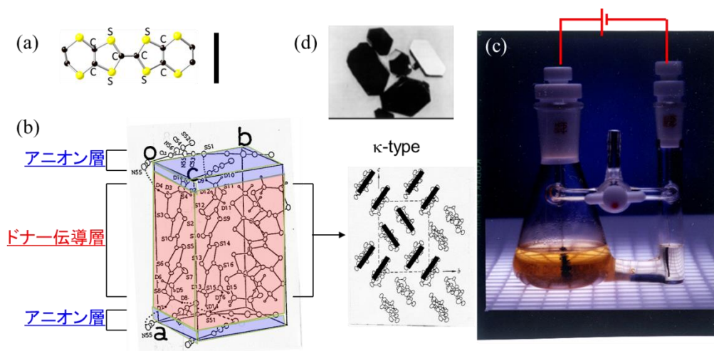
図 4 有機超伝導体 \kappa\text{-(BEDT-TTF)}_2\text{Cu(NCS)}_2 の(a) BEDT-TTF 分子、(b) 2 次元層状構造と伝導層内の \kappa 型ドナー配列、(c) 化学的電気酸化法による結晶育成風景と、(d) 得られた黒色単結晶。[3]
