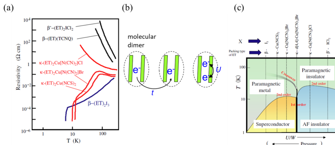
図 5 (a) \kappa-(\text{BEDT-TTF})_2\text{X} 等の電気抵抗率の温度依存性と (b) 統一的相図 [3,4]。
