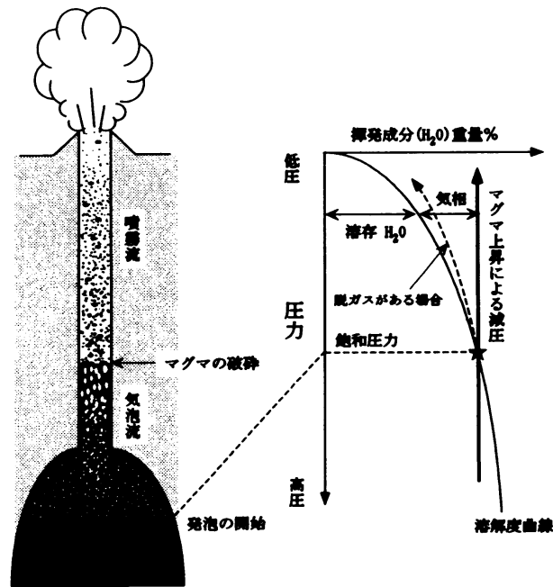
図 1: マグマの上昇ダイナミックスの概要と溶解度曲線の関係
