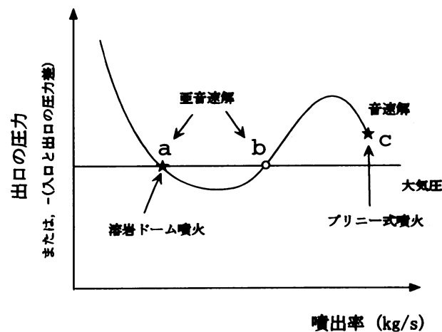
図 2: 多孔質媒体の火道中を上昇するマグマの定常流に関する噴出率と出口の圧力の関係の概念図
