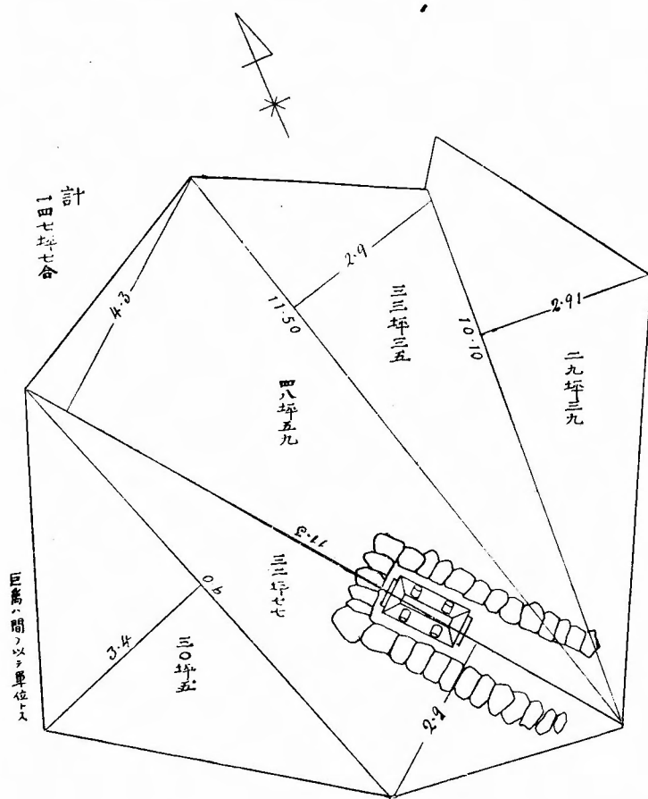
(Fig. 3) 第三圖 石室及石棺實測圖
