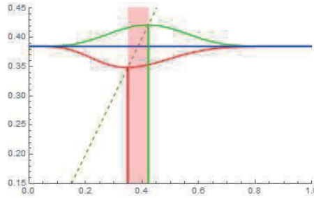
Figure 3: \phi(x) と \psi(x) の不動点と p_1, p_3 の事後推定区間 [0.349, 0.421]
