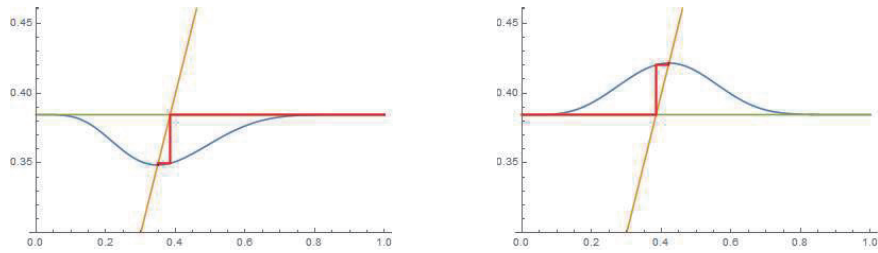
Figure 2: \phi(x), \psi(x) と反復によって得られる点列 x_n, y_n の軌跡の例
