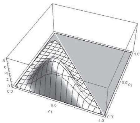
Figure 1: p = (p_1, p_2, p_3) のディリクレ分布の密度関数の例
