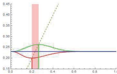
Figure 4: \phi(x) と \psi(x) の不動点と p_2 の事後推定区間 [0.201, 0.263]
