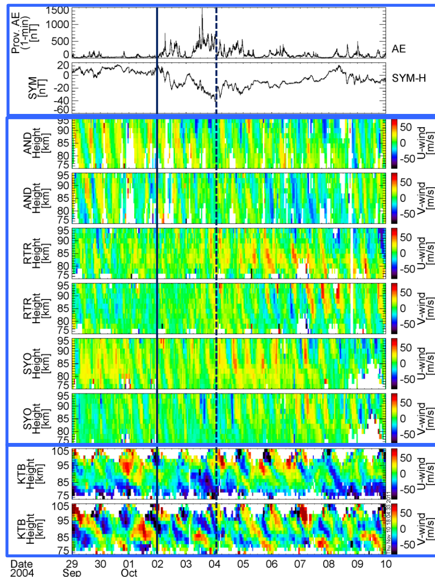
地磁気擾乱(2004年10月)時における風速変動
