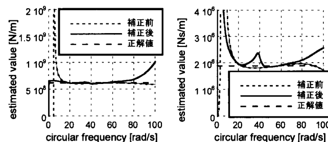
図8 剛性の同定 (4層)
