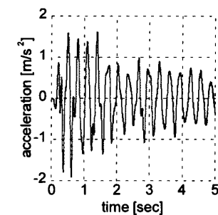
図3 出力データ (4層)
