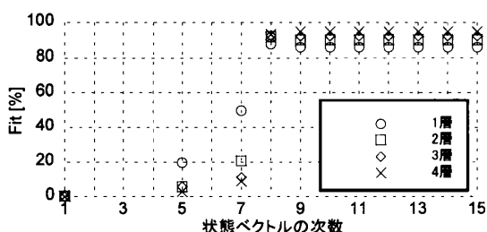
図4 状態ベクトルの次数とFitの関係
