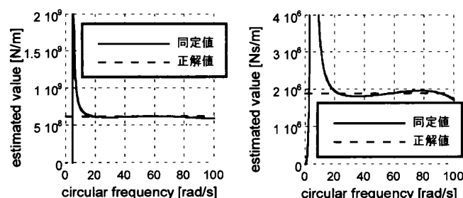
図5 剛性の同定 (4層)
