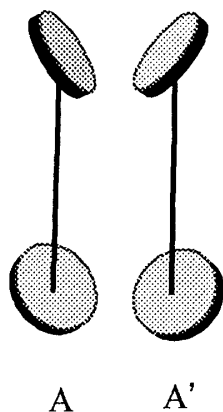
図 1: 粒子モデル
