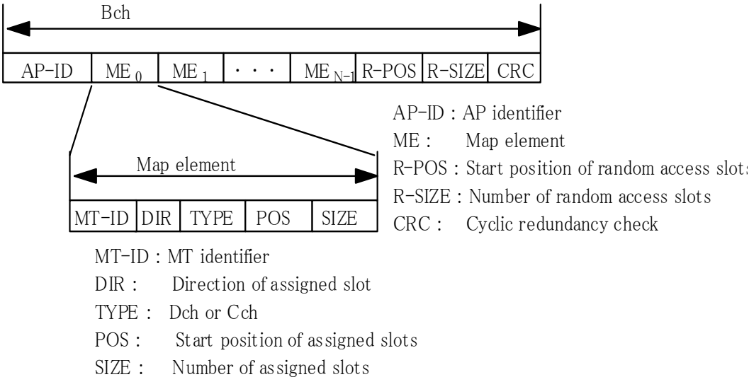
Fig. 3-3. Bch format.
