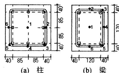
図2 断面形状
