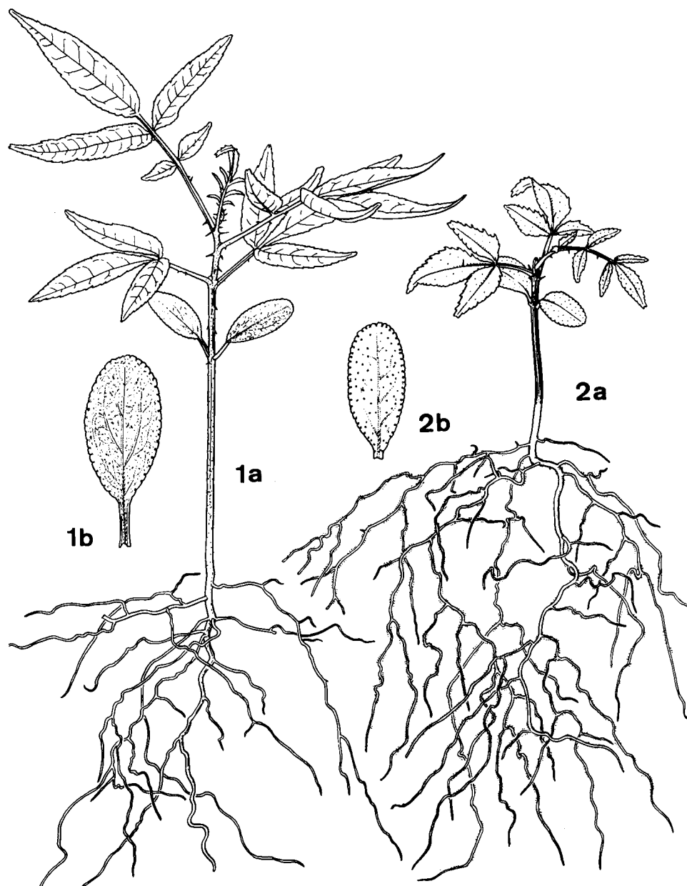
図-6 1. カラスザンショウ Zanthoxylum ailanthoides , 1a: habit (×1), 1b: cotyledon (×2)
