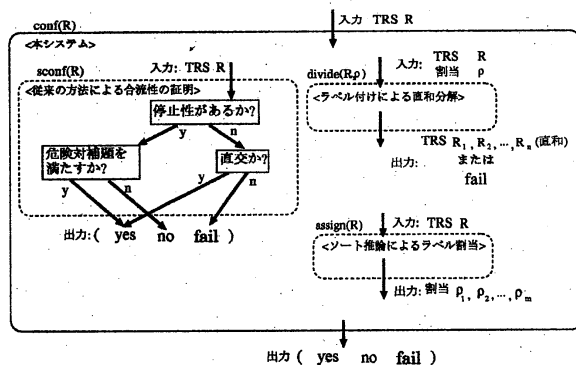
図 5.1: 合流性判定ツール
