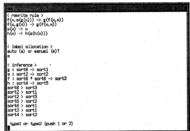
図 5.3: 順序ソート付きシグニチャ推論
