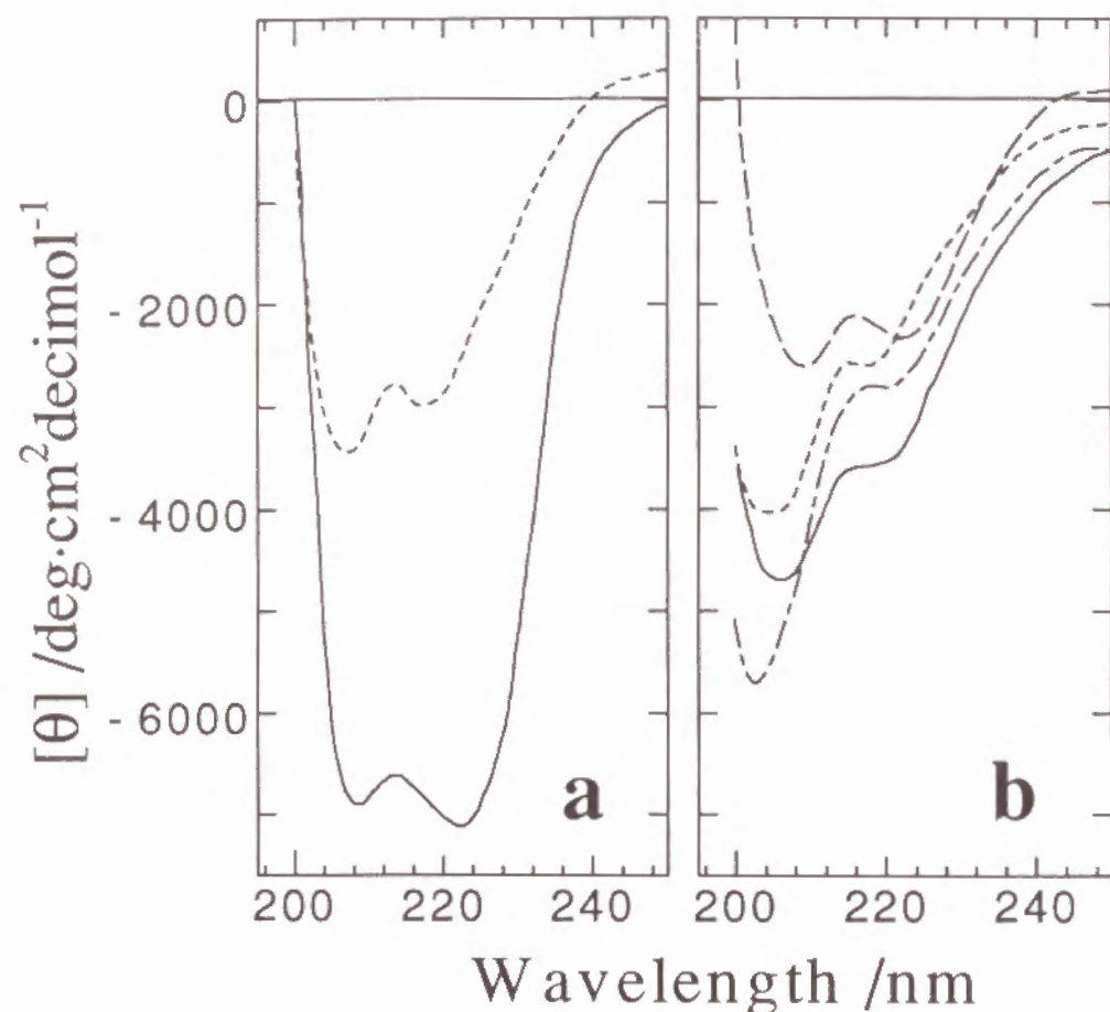
Figure 4. Circular dichroism spectra of (a) AMPA (—), DES3 (-----), (b) Nap-AMPA (----), Ant-AMPA (-----), AzoF-AMPA in the cis form (—), and AzoF-AMPA in the trans form (-----) in Tris-HCl buffer (10 mM, pH 7.8) at a concentration of 1.13 \mu M.
