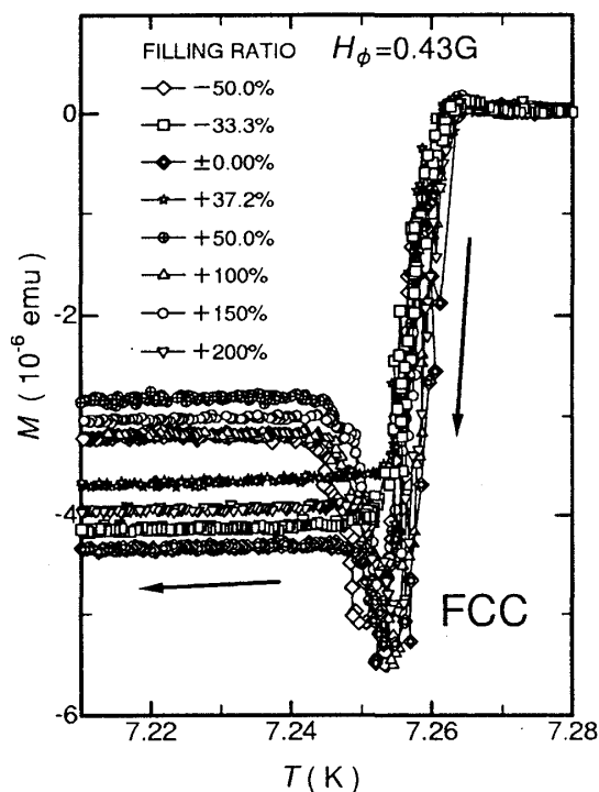
図 3: T_c 近傍の超伝導微細孔格子の磁化の温度依存
