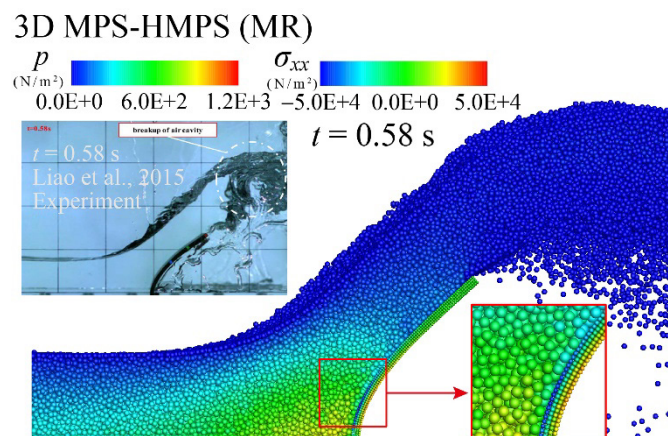
図4 解像度可変型三次元MPS-HMPSによるダムブレイクシミュレーション
