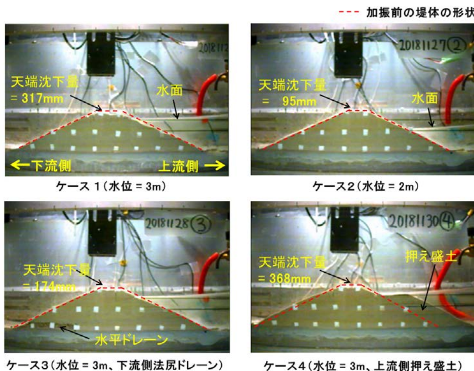
図2 たため池堤体の遠心力载荷装置を用いた模型実験
