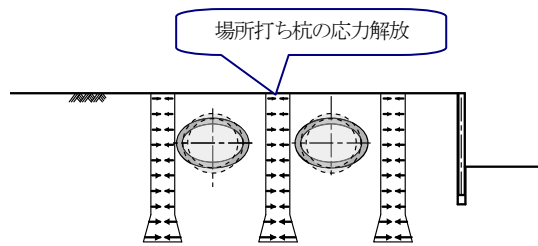
図-7 掘削中の課題(⑤杭打設)
