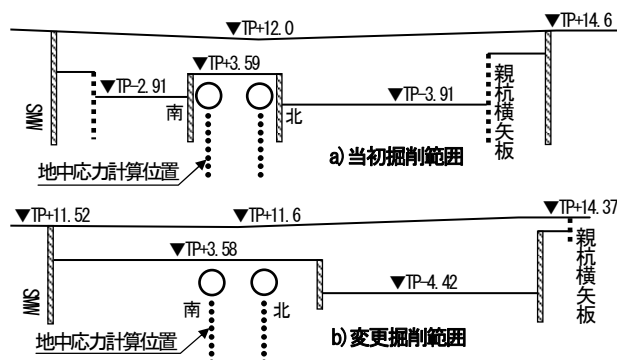
図-10 掘削断面形状の比較
