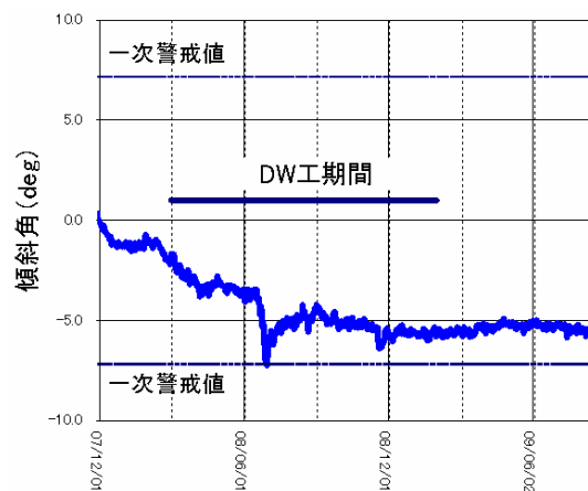
d) 傾斜角 (水準狂い)
