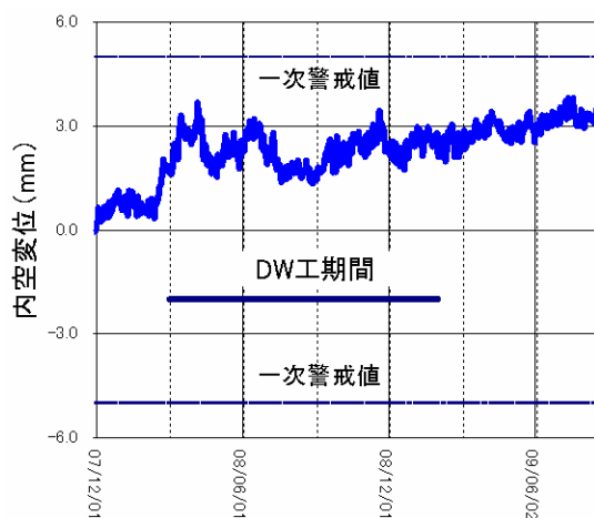
c) 内空変位 (SL)
