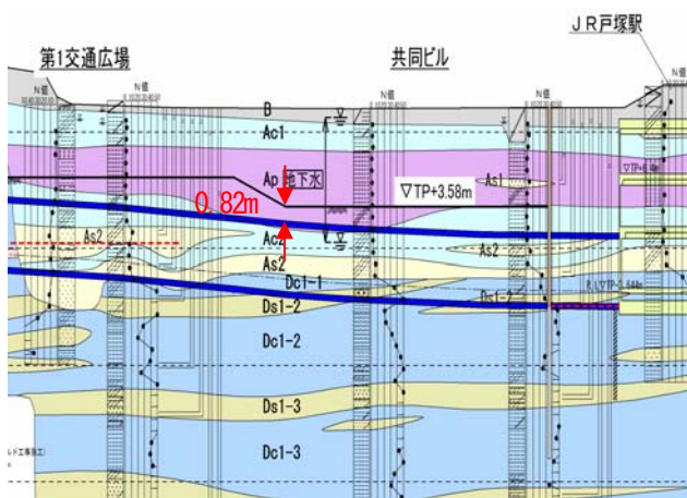
図-2 地質縦断面図
