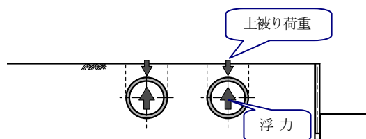
図-3 掘削中の課題（①浮力）
