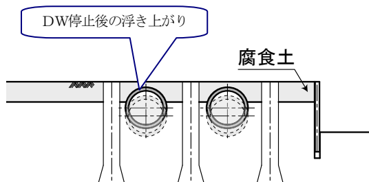
図-8 完成後の課題(腐植土層の圧密)
