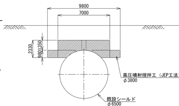
図-12 揚圧力対策工
