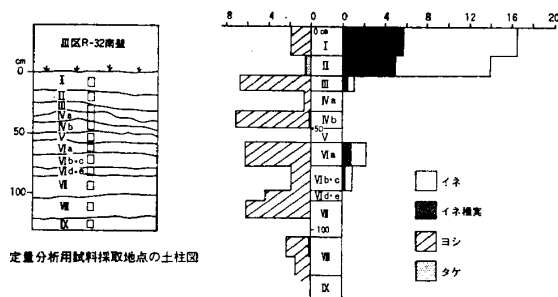
図4 垂柳遺跡（Ⅲ区 R-32 南壁）におけるイネ科植物生産量の推定（層位欄左の数字（cm）は地表面からの深さを示す）
