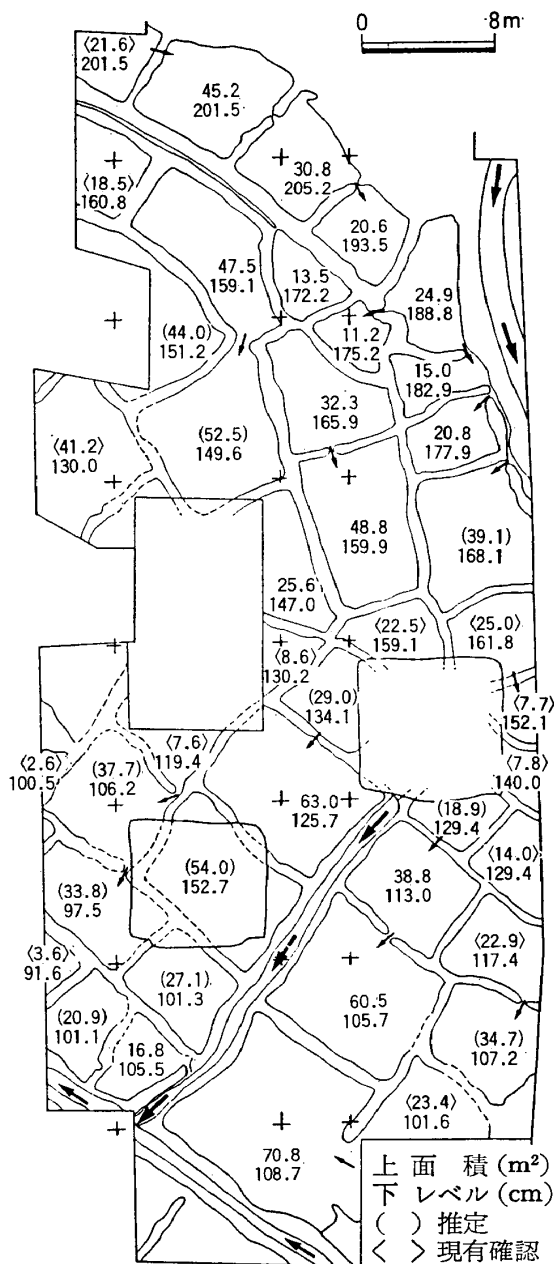
図3 目久美遺跡弥生時代中期（第1水田）の水田遺構（米子市教育委員会他 [1986] より引用）
