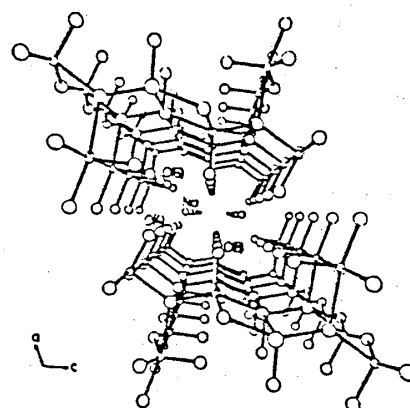
\beta\text{-Na}_x\text{V}_2\text{O}_5 の b 軸方向から見た鳥観図
