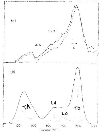
図1. ラマン散乱から導かれた \alpha\text{-Si} のフォノンDOS (a) と c-Si のDOS にもとづく解析 (b) 3
