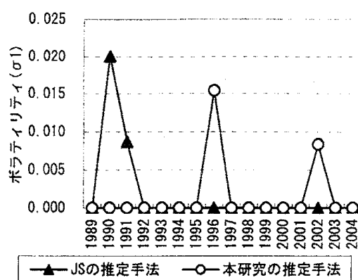
Fig.8 : Volatility parameters \sigma_1
