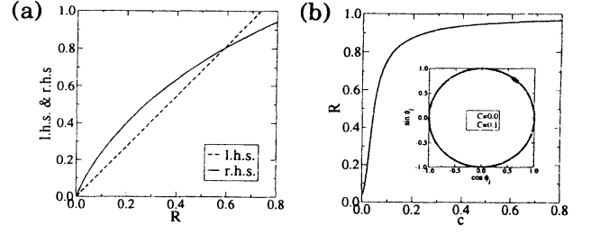
図3 (a) 自己無撞着な解析。自己無撞着条件の左辺と右辺が R > 0 で交われば、集団同期転移を示す。(b) スケールフリーネットワーク上の蔵本モデルの集団同期転移。結合強度 c と共に秩序パラメータ R が増大。挿入図は転移前 ( c = 0 ) と転移後 ( c = 0.1 ) での単位円上の振動子の分布。
