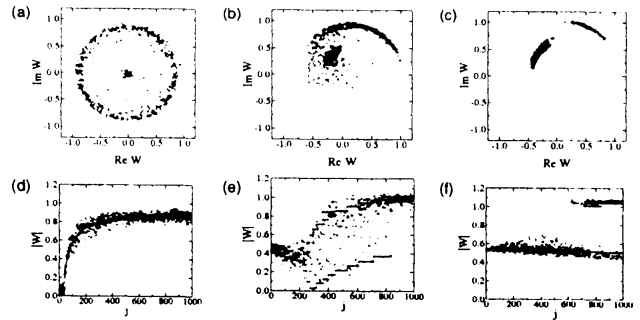
図5 スケールフリーネットワーク上の CGL モデルのダイナミクス (動的定常状態におけるスナップショット). (a,d) 部分振幅停止状態 ( K = 0.02 ), (b,e) カオス状態 ( K = 0.04 ), (c,f) クラスター状態 ( K = 0.08 ). (a),(b),(c) は全ての振動子の複素振幅 \{W_j\} の分布, (d),(e),(f) は振動子間の複素振幅の大きさ |W_j| をノード番号 j に対して表示. (d),(e),(f) の実線は平均場近似によるもの.
