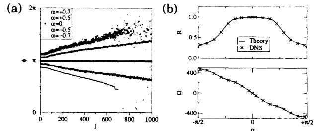
図4 ランダムスケールフリーネットワーク上の位相波. (a) 定常状態でのスナップショット. 横軸はノード番号 (次数の大きい順にソート). \omega = 1.0 , c = 5.0 , N = 1000 , \langle k \rangle = 20 で、いくつかの \alpha の値について表示. (b) 自己無撞着理論により得られた集団振動の振幅 R と振動数 \Omega を直接数値計算により得られた値と比較. 横軸は \alpha で、 \alpha = 0 の時 \Omega = 0 となるように位相を定義している.
