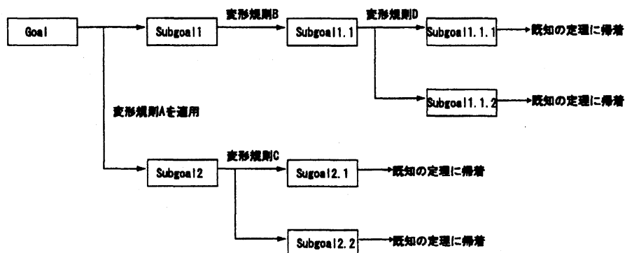
図 2: 証明の流れの概念図
