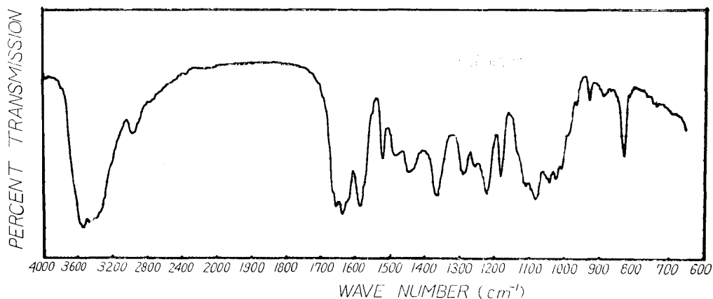
Fig. 2 IR spectrum of haplormosin
