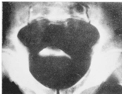
第5図 20%NaJ30cc+空気 100cc 排除後空気 100cc 注入時 (造影剤残存による陰性結石像をみる)
