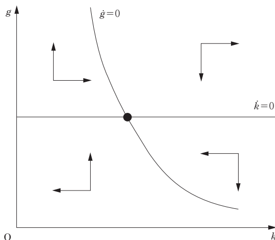
図2 長期カレツキアン・モデルの動学
