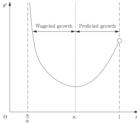
図1 利潤シェアと短期均衡における資本蓄積率の関係 ( f(1) > 0 のケース)
