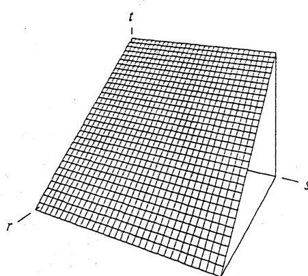
F_N: r+t < 1, s < 1
