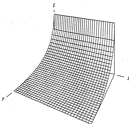
F_R: \sqrt{r} + \sqrt{t} < 1, s < 1
