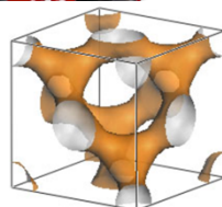
電子構造
