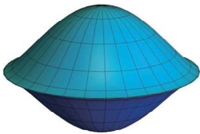
図 3: n = 2 , K = 2/3 の場合の f_k の図 (例 2.10).
