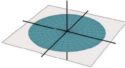
図 4: \mathbf{R}^3 内の f(S^2) の図 (例 3.1).
