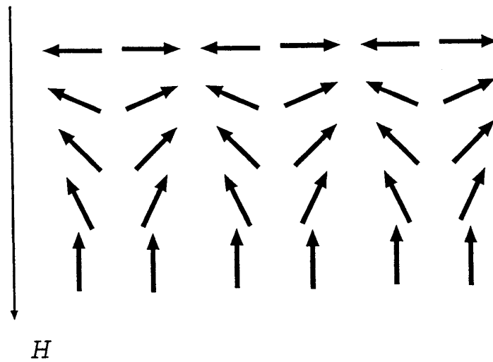
Figure 3: 古典的反強磁性体の磁化過程。スピンの磁場の方向に傾く角度が磁場 H の増加とともに連続的に変化する。
