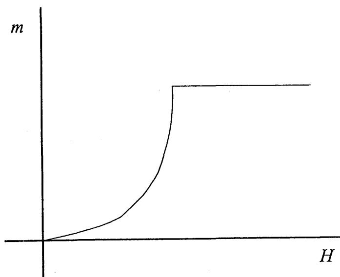
Figure 2: 典型的な磁化曲線。磁場 H の増加とともにめらかに増加する。
