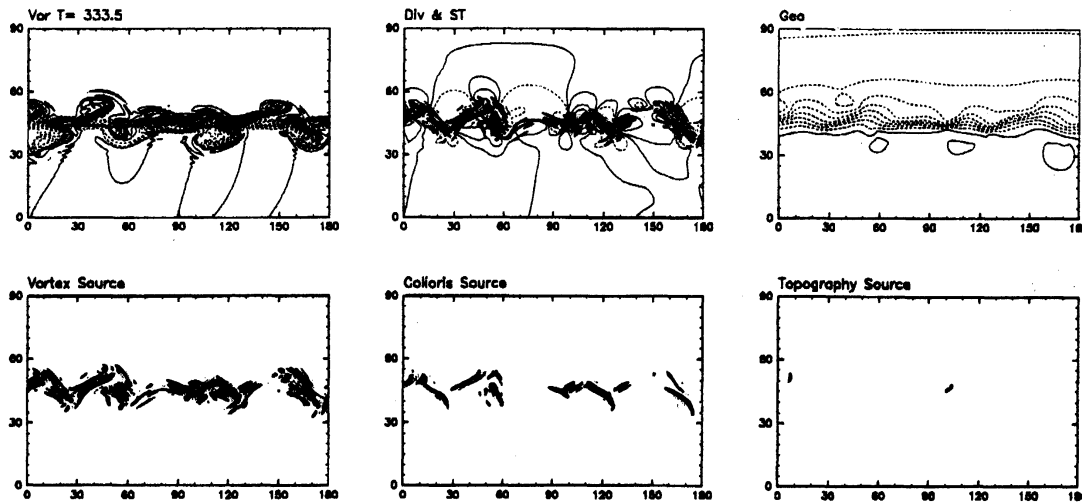
図 4: 流れ場と重力波ソース (上段) 及び重力波ソースの各項 (下段) のスナップショット. 縦軸は緯度, 横軸は経度で, 北半球の半面を拡大して示す. (左上) 渦度, (中上) 発散と重力波ソース (式 (10) の右辺), (右上) ジオポテンシャルハイト, (左下) 渦によるソース (右辺第 1 項), (中下) 地球回転に関わるソース (右辺第 2 項), (右下) 水深の変化によるソース (右辺第 3 項) である. 重力波ソースはトーンで示され, 上段における, コンターの値及び意味は (左上) が 5 \times 10^{-5} 間隔であることを除いて, 図 3 と同様である.
