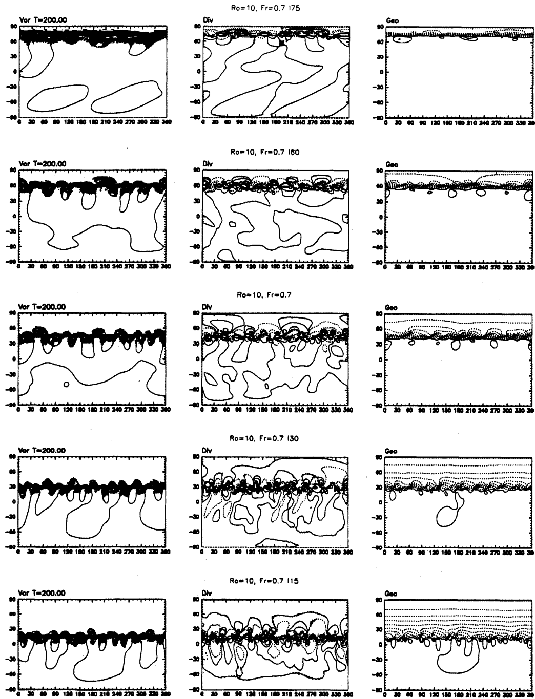
図 6: 流れ場のジェットの緯度依存性. 上からそれぞれジェットの緯度が 75, 60, 45, 30, 15 で, (左) 渦度, (中) 発散, (右) ジオポテンシャルある. 縦軸は緯度, 横軸は経度である. ジェットの中心緯度は, コンター及びハッチの値及び意味は図 4 と同様である.
