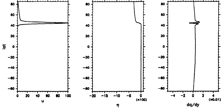
図 1: Ro = 10 , Fr = 0.7 における帯状な基本場の緯度構造の拡大図: (左) u(\theta) , (中) \eta(\theta) , (右) d\bar{q}(\theta)/d\theta .
