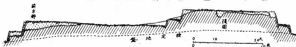
(Fig. 11) 第十圖 姫塚復原縦断面圖
