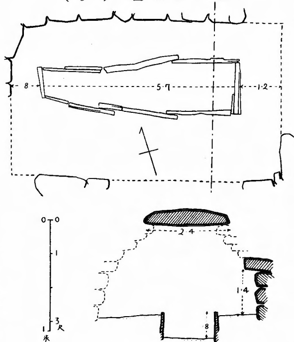
摺鉢谷一石塚石室實測圖
