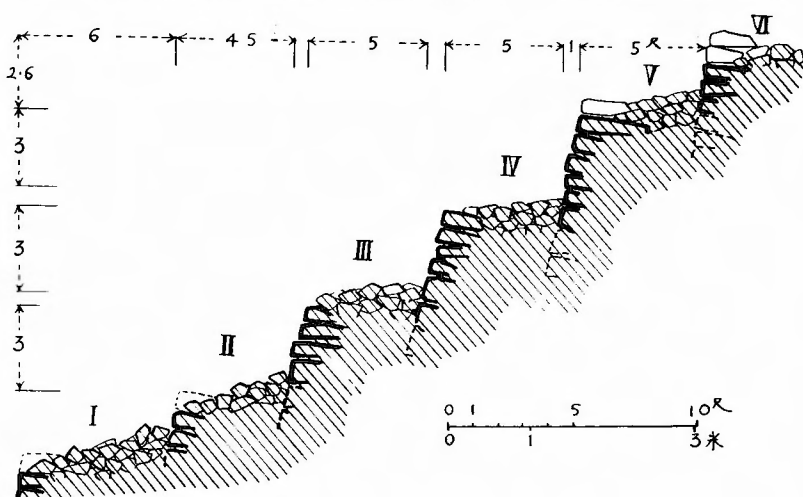
第 二 十 二 圖 稻 荷 山 姫 塚 前 方 石 築 狀 態 (斷 面 圖) (Fig. 22)
