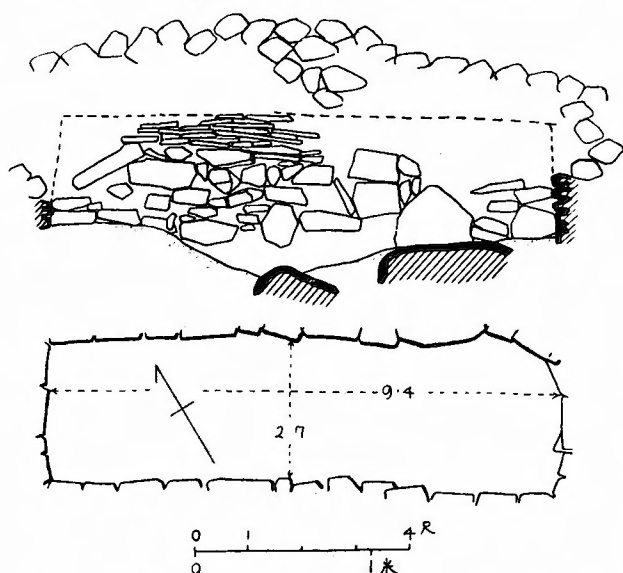
第 十二 圖 西北端石塚の石室 (Fig. 20)
