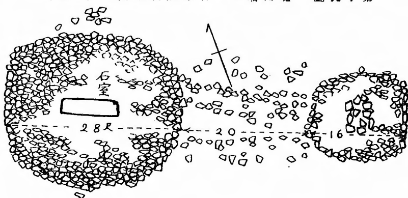
(Fig. 19) 圖略狀形塚石一の端西北 圖九十第
