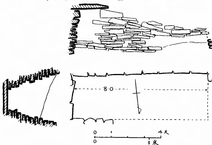
猫塚中央部第一石室圖
