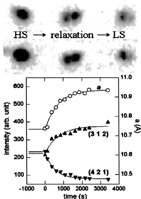
図7．鉄系スピクロスオーバー錯体 [\text{Fe}(\text{2-picolyamine})_3]\text{Cl}_2\text{EtOH} の光誘起相の緩和過程。高スピン (HS) 相と低スピン (LS) 相の共存が観測された。
