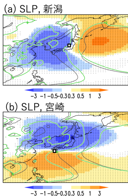
図4：新潟と宮崎の極端高温事例の SLP の平年偏差。点は偏差が統計的に有意な箇所。(Ito et al. 2022 から引用、一部変更)
