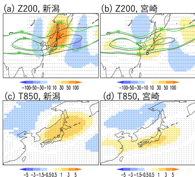
図3：新潟と宮崎の極端高温事例の (a, b) Z200 (m) と (c, d) T850 (K) の平年偏差。点は偏差が統計的に有意な箇所。(a, b) コンターは東西風速で、緑が極端高温事例、黒が平年値。(Ito et al. 2022 から引用、一部変更)
